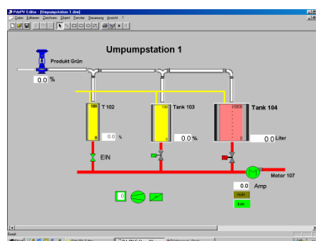
Bild 4. Prozessbild-Generator
